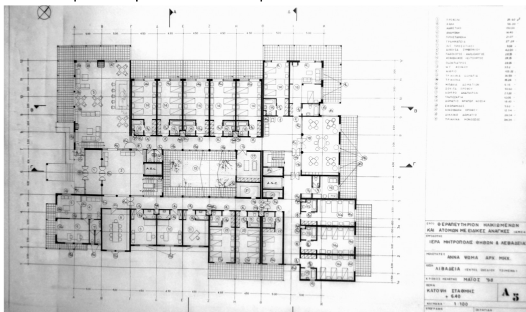
Εικ. 4. Κάτοψη στάθμης + 6.40 από το επίπεδο του εδάφους και συν 1,00 μ από τη στάθμη της οδού
