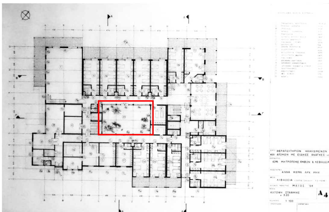
Εικ. 5. Κάτοψη στάθμης + 3.20 από το επίπεδο του εδάφους
