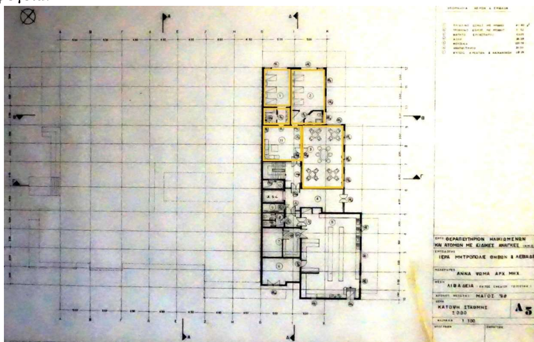
Εικ. 6. Κάτοψη στη στάθμη ± 0.00 (στο επίπεδο του εδάφους)
